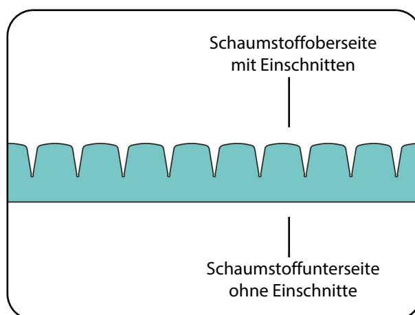
Abb. 6.1.01 - Querschnitt-Würfelstruktur
