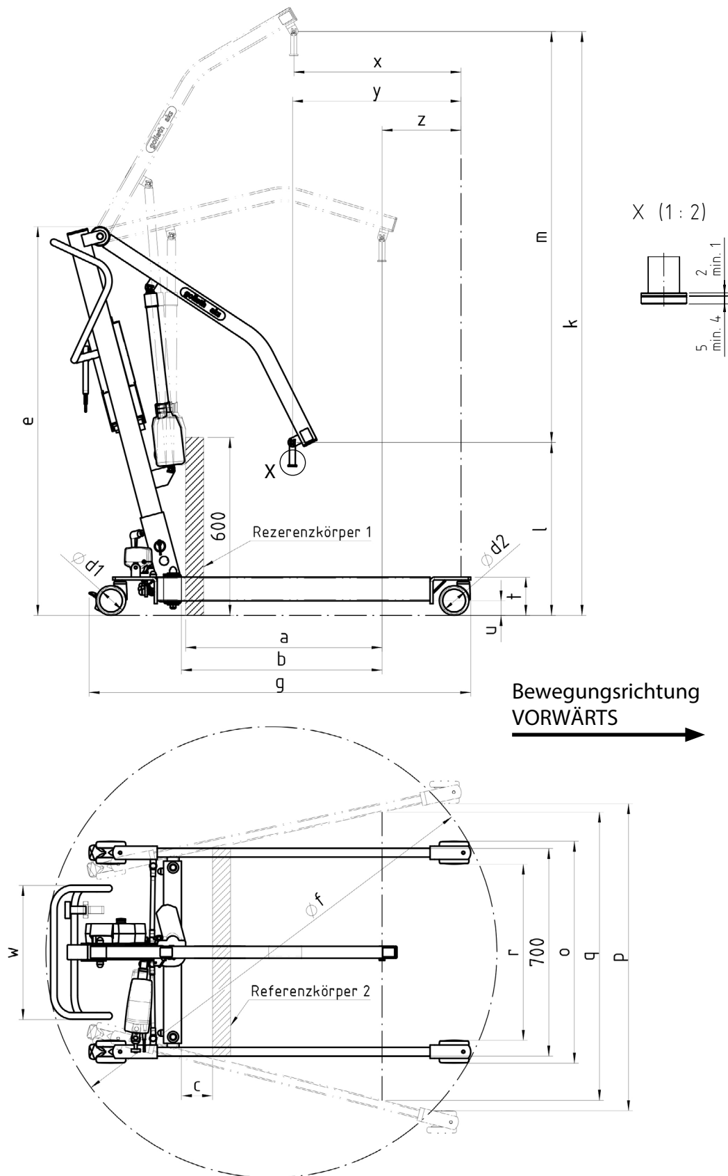
Abb. 21.01 – goliath® - Maßskizze Abmessungen (L x B x H): 1.285 x 745 x 1.310
