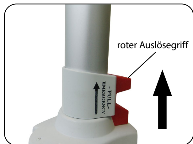
Abb. 8.6.02 - mechanische Notabsenkung
