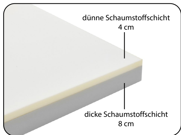
Abb. 6.1.01 - Schaumstoffschichten (Bsp. aks-duoplot)
