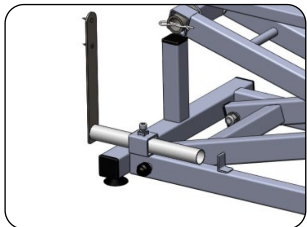
Abb. 6.1.09 – Abstandswinkel befestigen
