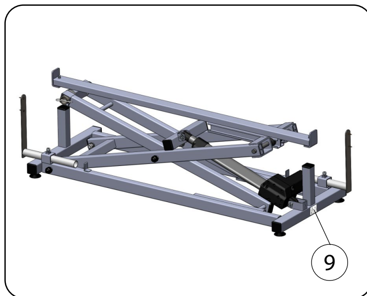
Abb. 20.03 – Scherehub
