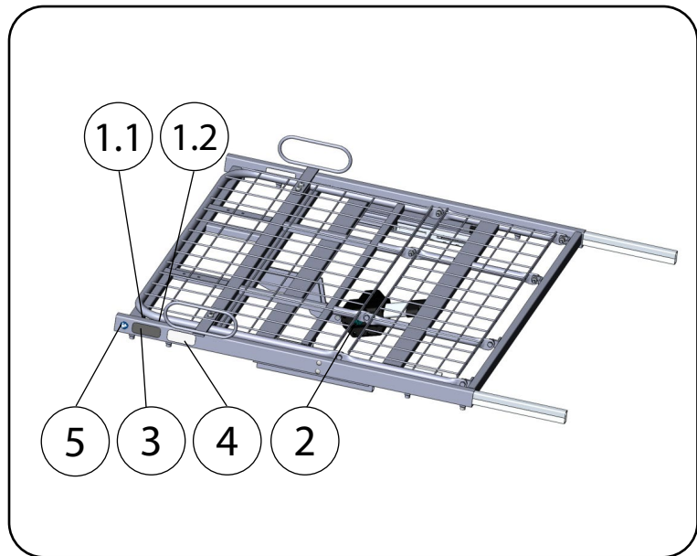
Abb. 20.02 – Fußauflage
